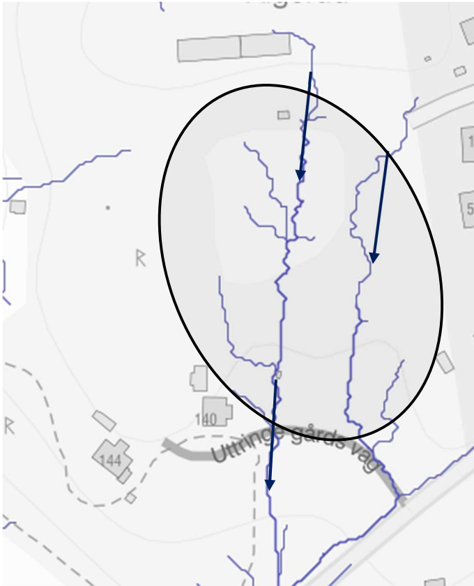
Figur 9. Avrinningsvägar, Uttringe 1:90, (blåa pilar) vid 44 mm regn efter nationella höjddmodellen. Svart markering visar ungefärlig fastighet. (Scalgo Live, 2023)
