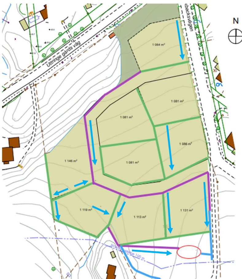
Figur 8. Förslag på dagvattenhantering för Uttringe 1:57. Grönt är regnbäddar (biofilter), Lila är nya makadamdiken och Blå är befintliga öppna diken. Blå pilar visar rinnvägar för avledning. Röd cirkel visar föreslagen damm.
