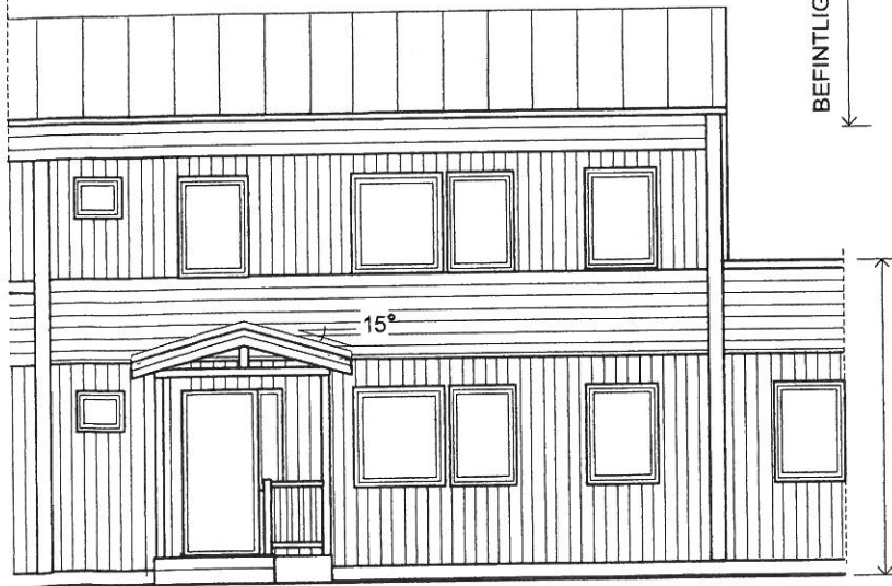
NY FASAD SKALA 1:100
