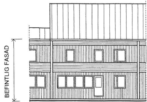
SKALA 1:200
