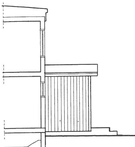
SEKTION/FASAD
