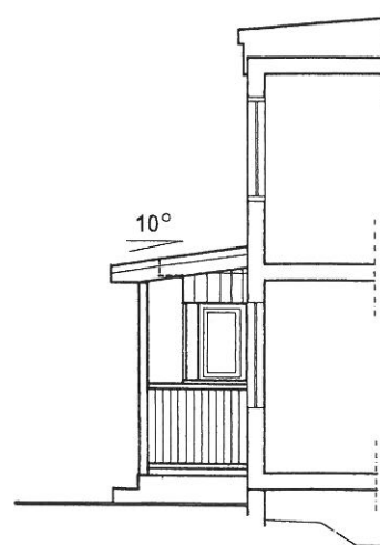
SEKTION/FASAD
