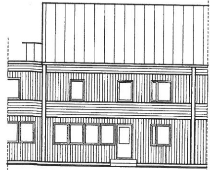
SKALA 1:200
