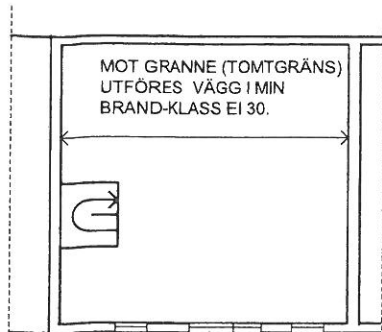
PÅBYGD VÅNINGSPÄN SKALA 1:200
