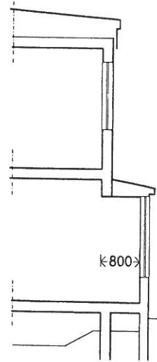
SEKTION
